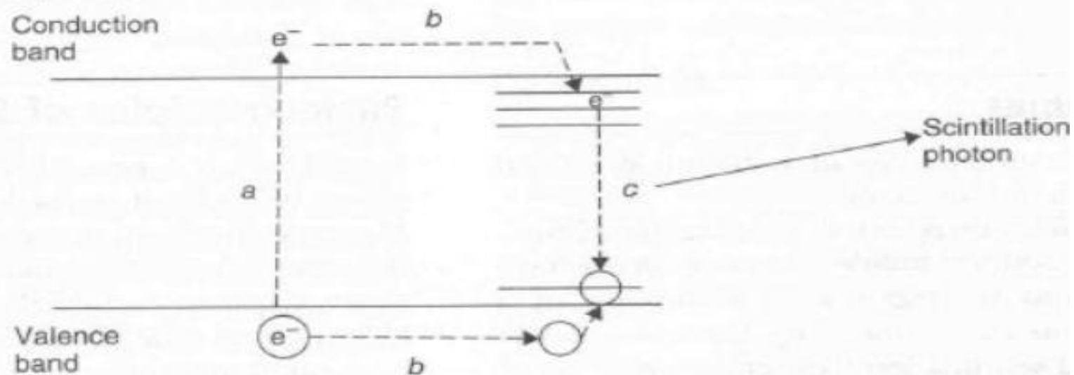
圖：碘化鈉（鉀）閃爍體晶體能帶示意圖
